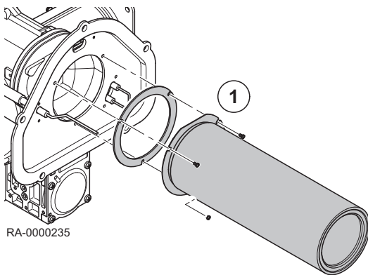
Fig.49 Retrait du tube brûleur
