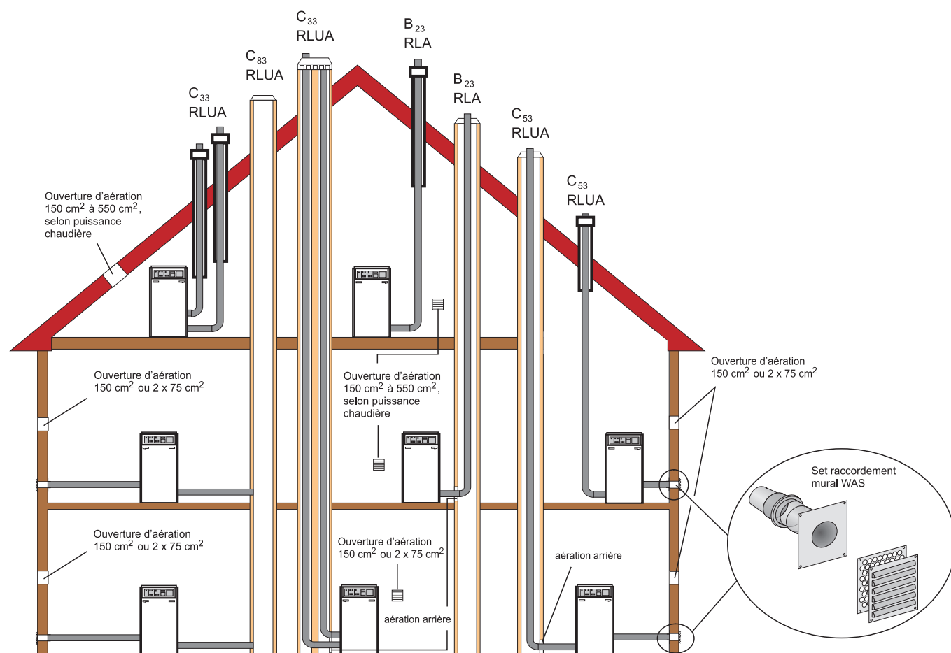
Fig.23 SGB avec fumisterie SAS pour fonctionnement dépendant de l'air ambiant et fonctionnement indépendant de l'air ambiant
