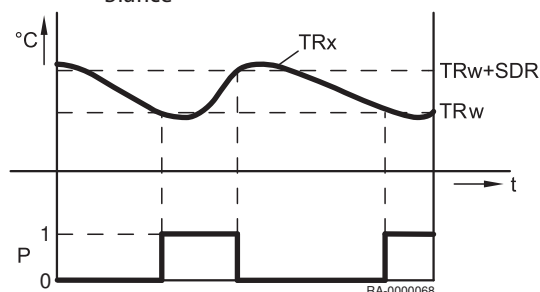
Fig.31 Limitation de la température d'ambiance
