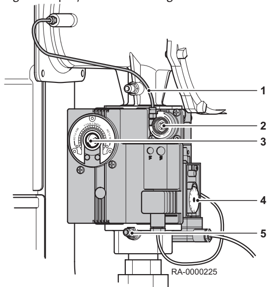
Fig.28 Aperçu de la vanne de gaz
