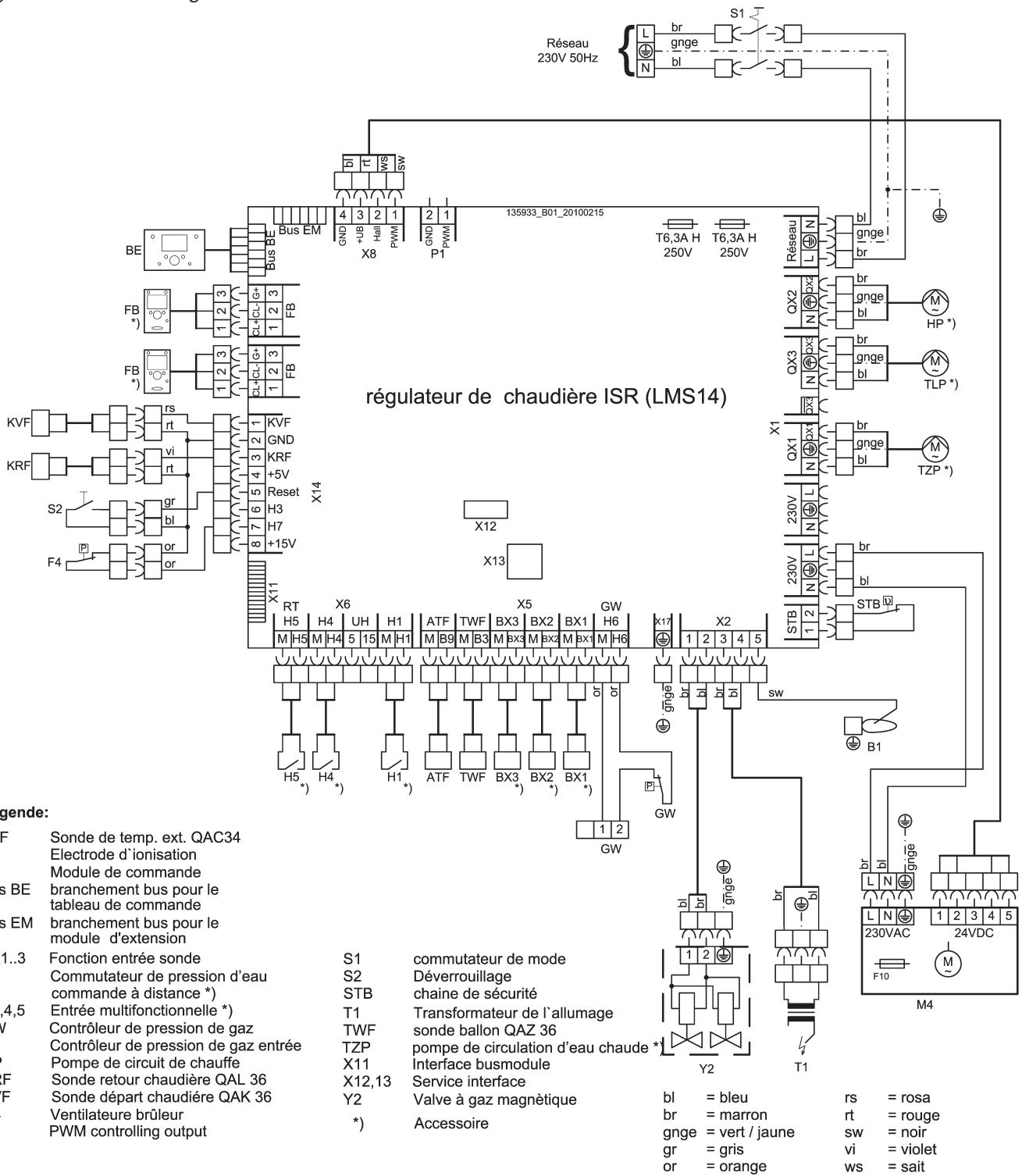
Fig.3 Schéma de câblage
