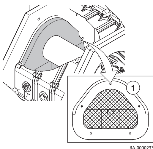
Fig.47 Position de l'isolation de la chambre de combustion.
