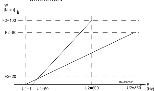
Fig.42 Exemple de deux courbes de capteur différentes
