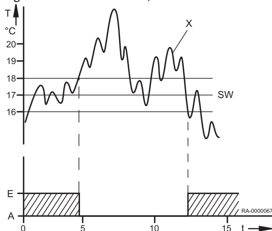
Fig.30 Limite chauffe été/hiver
