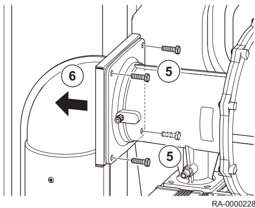
Fig.45 Desserrer le tuyau de raccordement gaz
