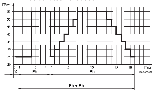
Fig.35 Profil de température de la fonction du durcissement de sol
