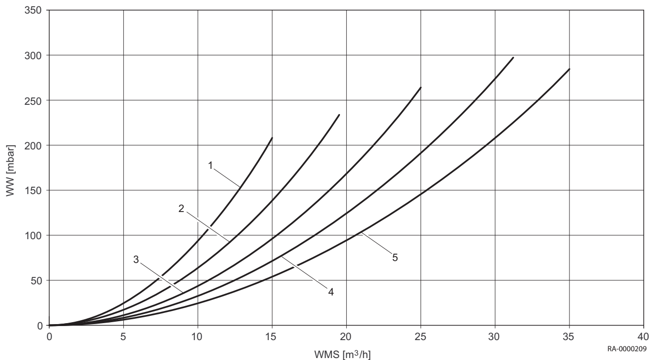
Fig.1 Chute de pression sur circuit secondaire
