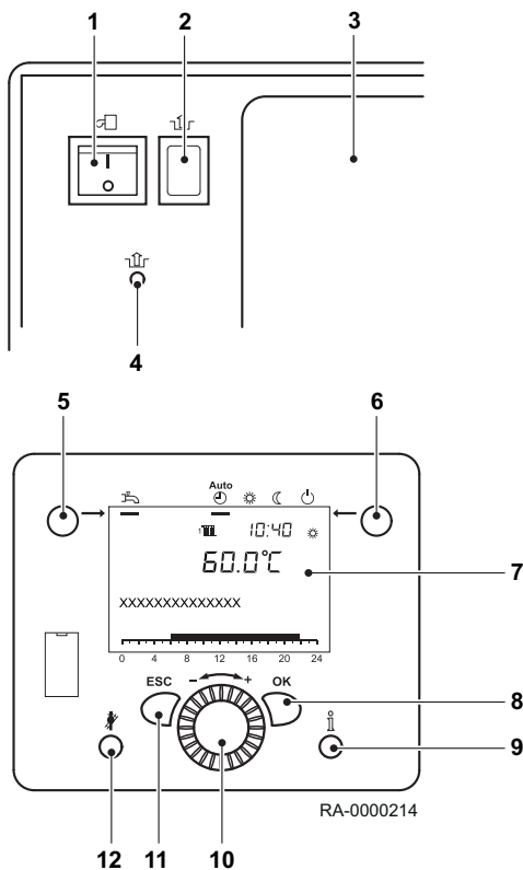
Fig.7 Éléments de fonctionnement
