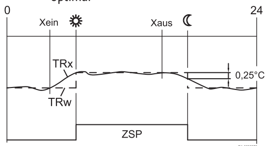
Fig.33 Commande de démarrage et d'arrêt optimal
