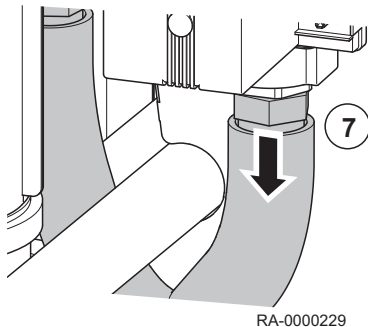
Fig.45 Desserrer le tuyau de raccordement gaz
