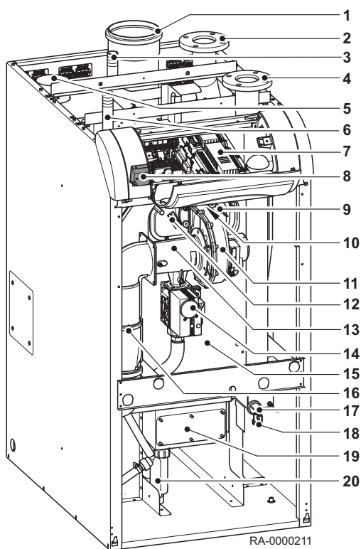
Fig.4 Vue d'ensemble de la chaudière SGB 125 H - 170 H
