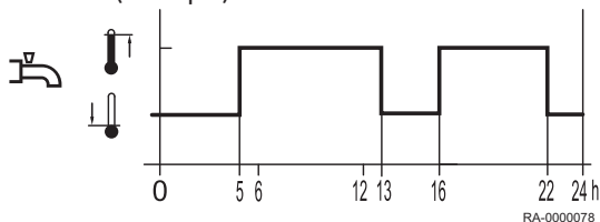
Fig.37 Déclenchement en fonction du programme de commutation de l'heure 4 (exemple)
