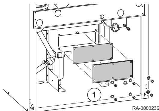
Fig.50 Retrait du couvercle du bac collecteur des fumées
