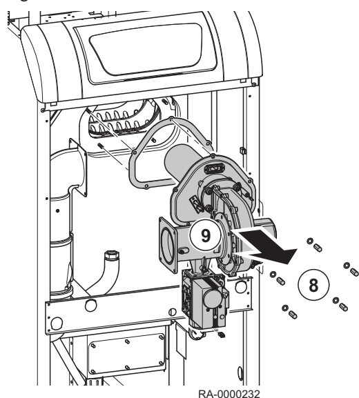
Fig.46 Démontez le brûleur
