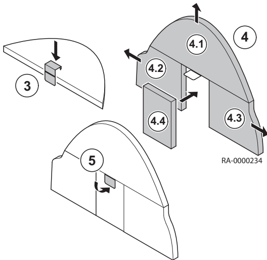
Fig.48 Insérer l'isolation de la chambre de combustion.
