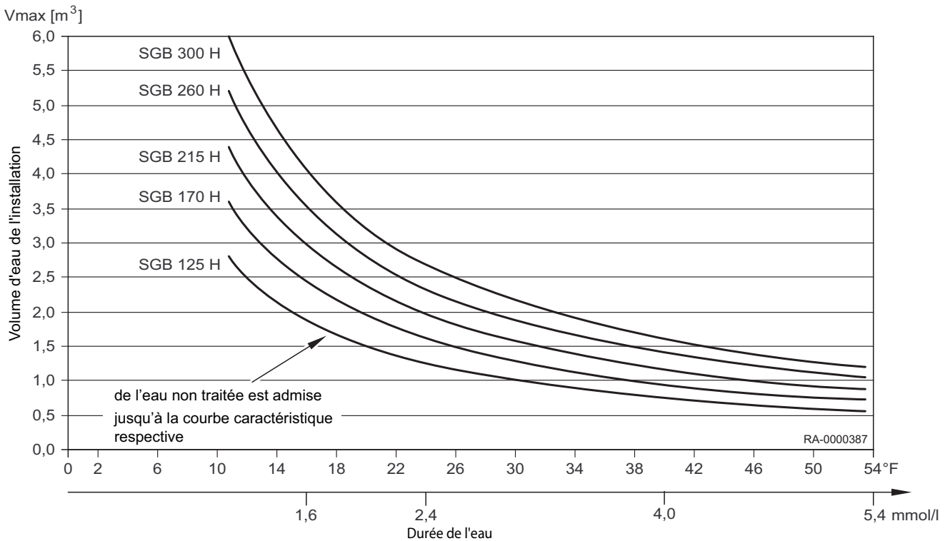
Fig.9 Diagramme de la dureté de l'eau
