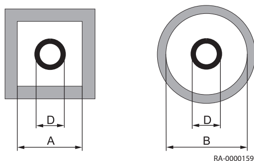
Fig.24 Dimensions minimales du conduit
