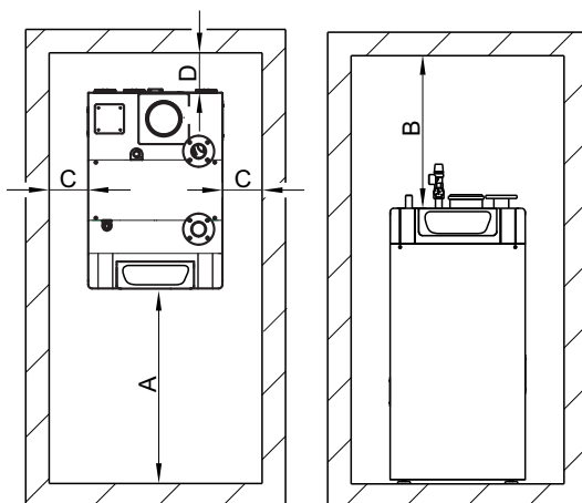
Fig.10 Espace nécessaire recommandé
