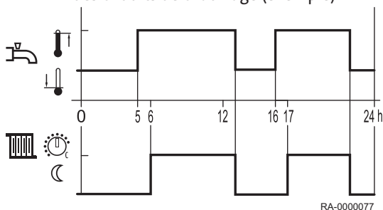
Fig.37 Déclenchement en fonction du programme de commutation de l'heure 4 (exemple)
