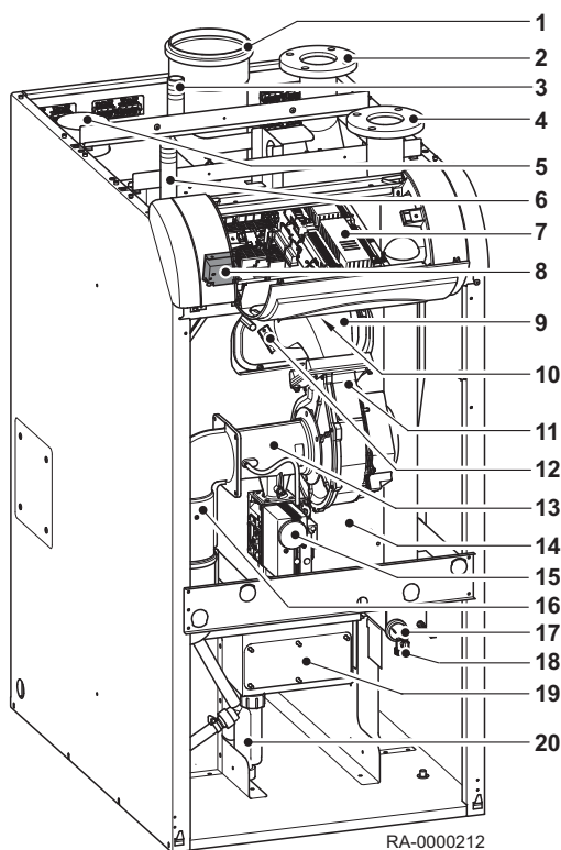
Fig.5 Vue d'ensemble de la chaudière SGB 215 H - 300 H
