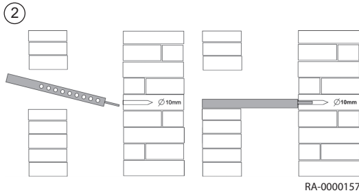
Fig.26 Insertion dans le conduit
