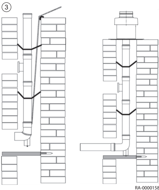
Fig.26 Insertion dans le conduit
