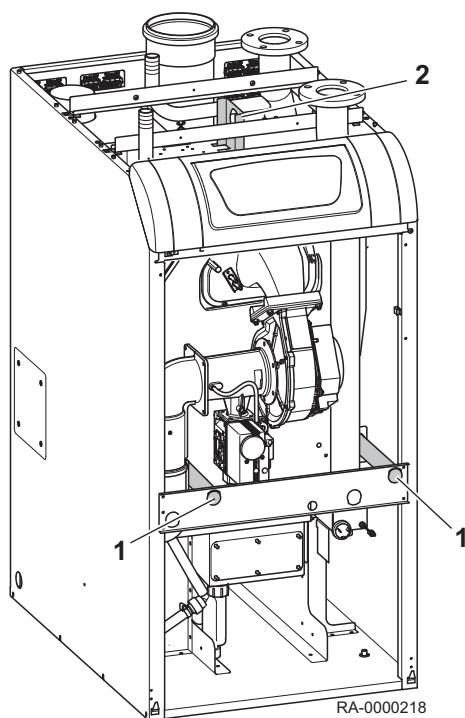
Fig.11 Équipement de transport
