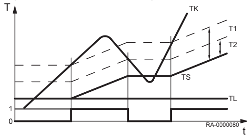
Fig.39 Commande de charge / schéma)
