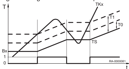
Fig.40 Chargement du ballon tampon
